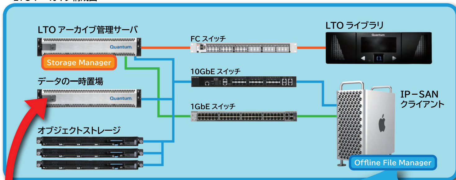
LTO アーカイブ構成図
